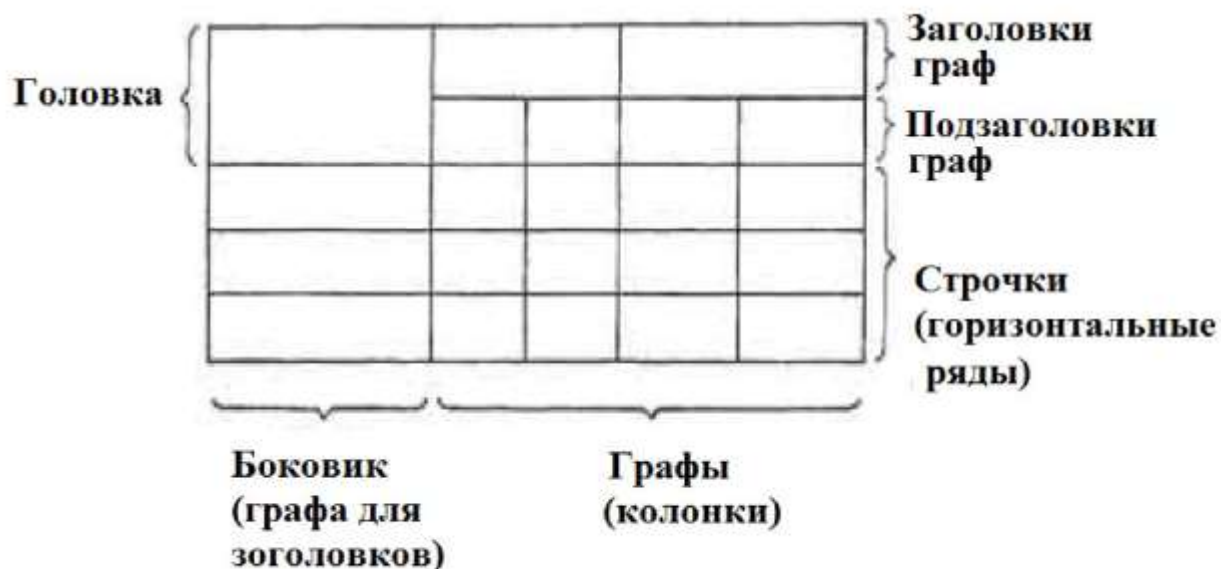
Рисунок 8.1 – Пример таблицы
